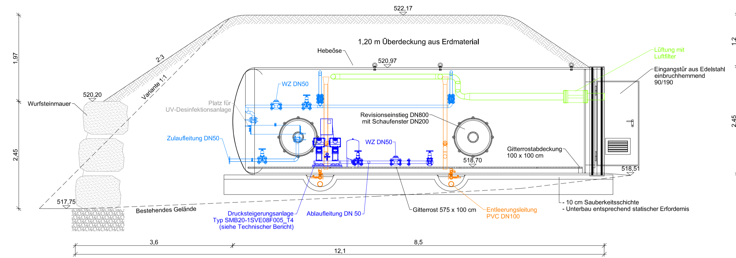
Schnitt A-A
