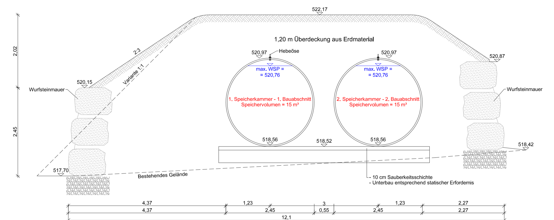
Schnitt C-C
