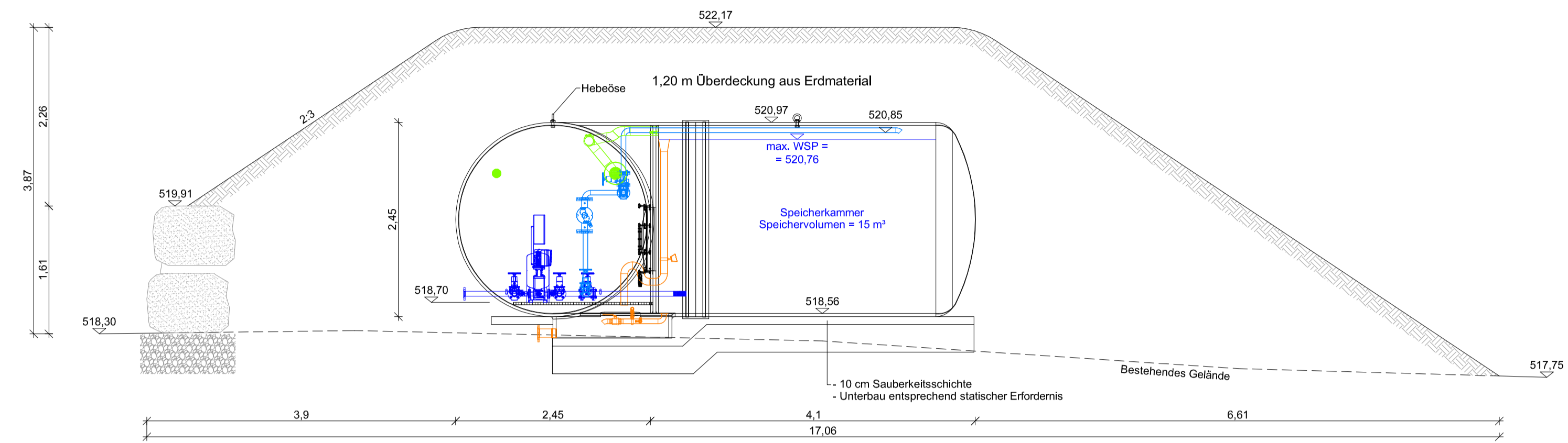
Schnitt B-B
